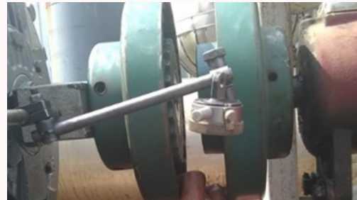
Alineación de Motor con Bomba de Sistema Chiller - Centro Comercial
